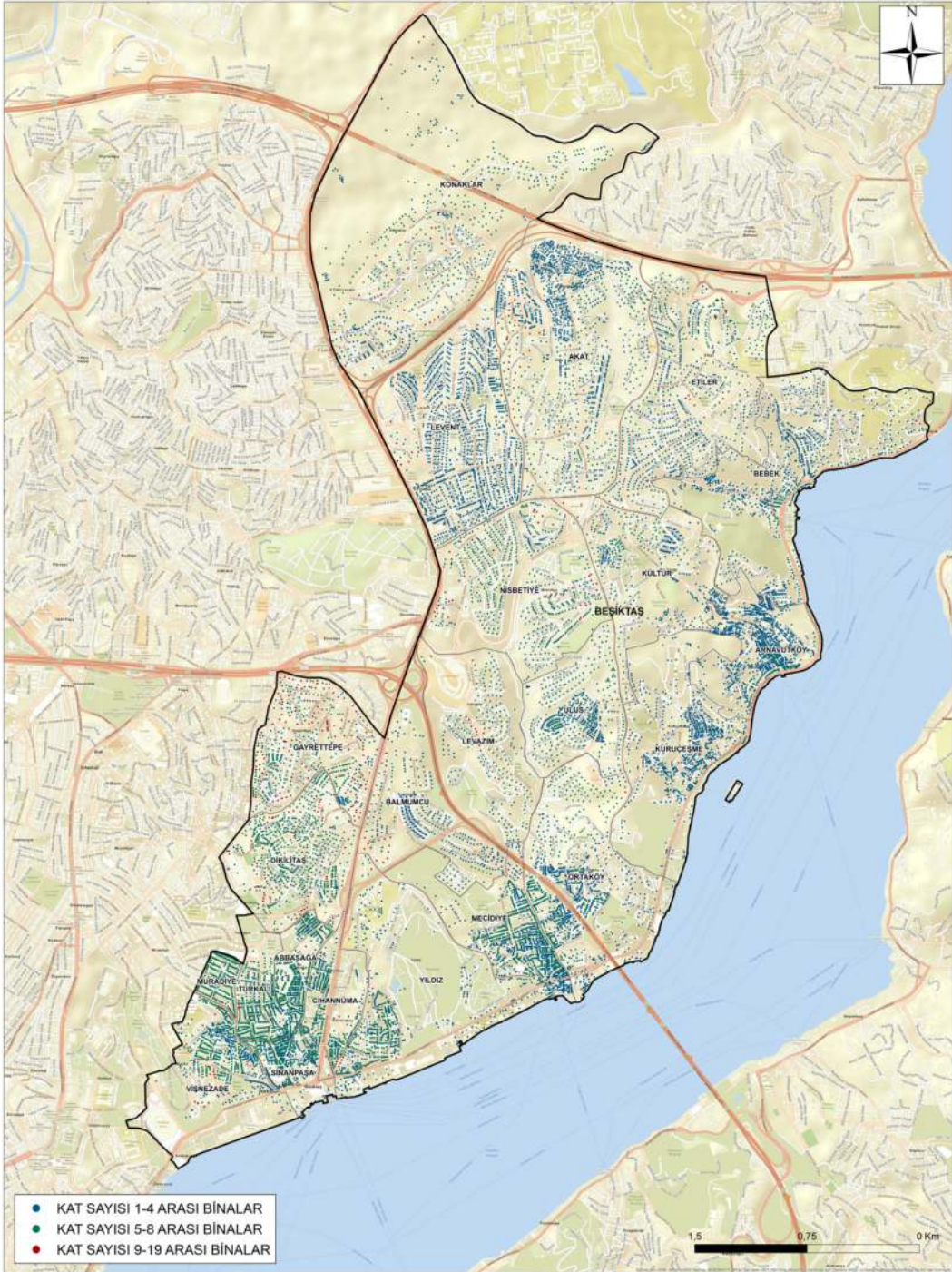
Şekil 3-6: Beşiktaş İlçesi Kat Sayısına Göre Bina Dağılımları
