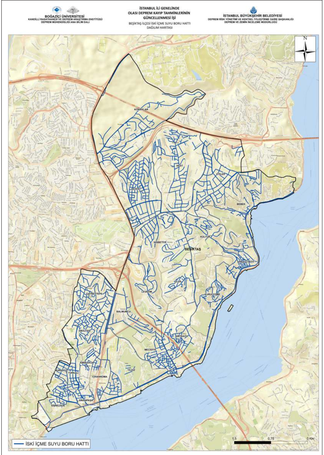
Şekil 3-10: Beşiktaş İlçesi İSKİ İçme Suyu Boru Hattı Dağılımları
