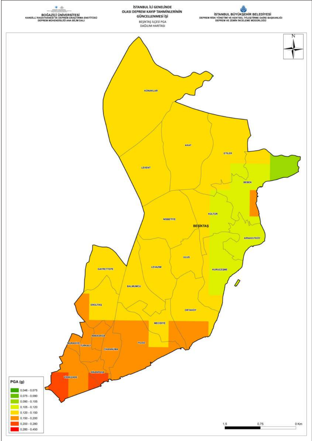
Şekil 4-4: Senaryo Depremi İçin Elde Edilen Beşiktaş İlçesi Zemin Bağımlı Medyan En Büyük Yer İvmesi (PGA) Dağılımı
