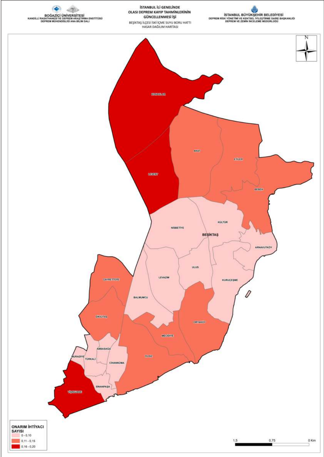
Şekil 5-12: Mw=7.5 Senaryo Depremi İçin Beşiktaş İlçesi İSKİ İçme Suyu Boru Hatları Tahmini Onarım İhtiyacı Dağılım Haritası
