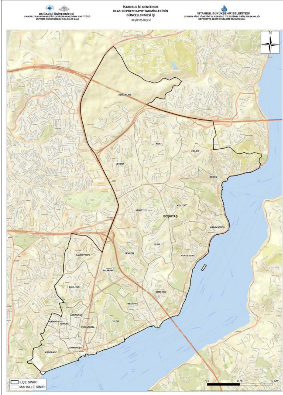
Şekil 3-1: Beşiktaş İlçesi ve Mahalleleri
