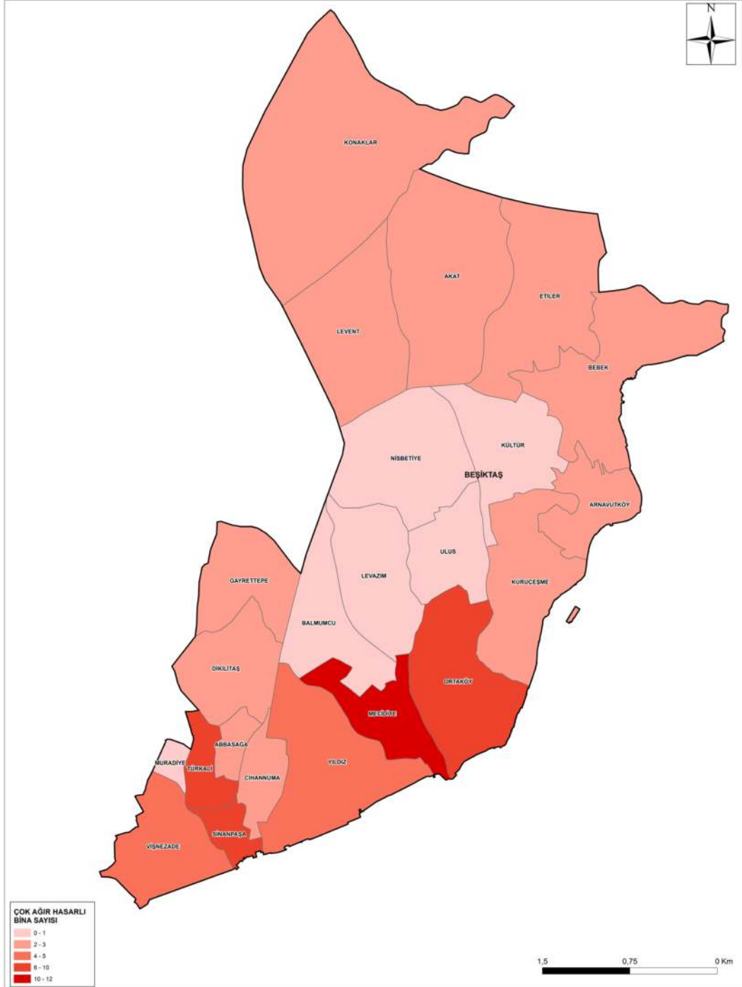
Şekil 5-2: Mw=7.5 Senaryo Depremi İçin Beşiktaş İlçesi Tahmini Çok Ağır Hasarlı Bina Sayısı Dağılım Haritası
