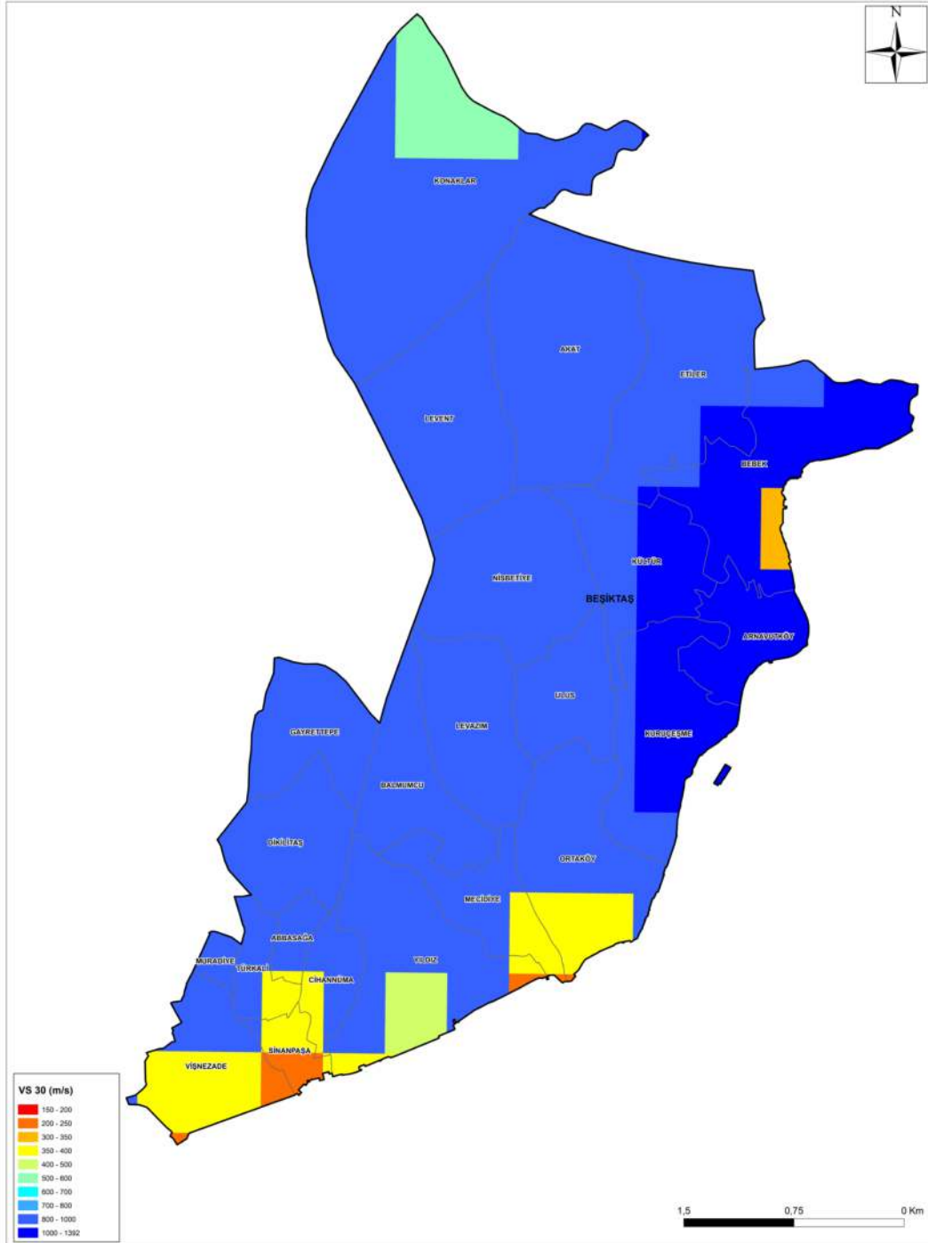
Şekil 4-1: Beşiktaş İlçesi V_{s30} Dağılımı
