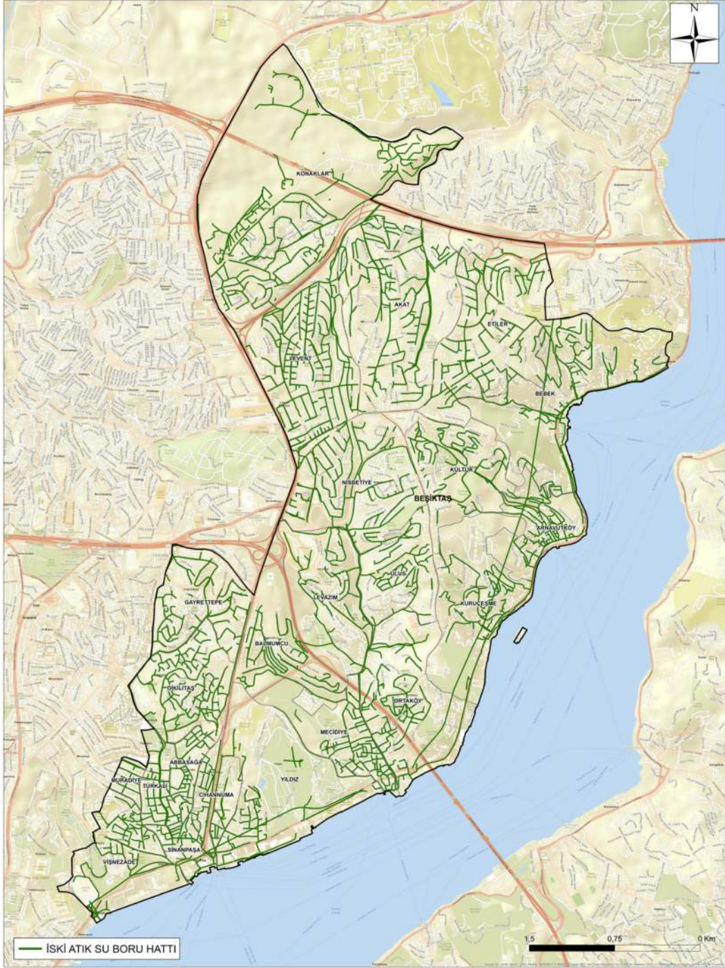
Şekil 3-11: Beşiktaş İlçesi İSKİ Atık Su Boru Hattı Dağılımları
