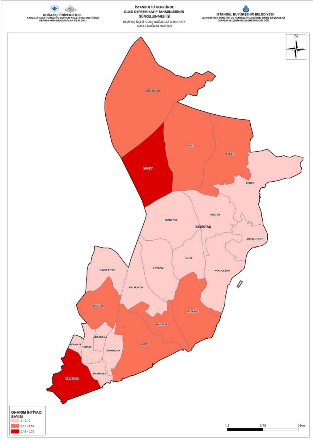
Şekil 5-10: Mw=7.5 Senaryo Depremi İçin Beşiktaş İlçesi Doğal Gaz Şebekesi Boru Hatları Tahmini Onarım İhtiyacı Dağılım Haritası
