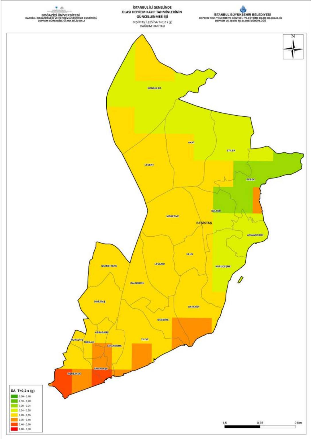
Şekil 4-6: Senaryo Depremi İçin Elde Edilen Beşiktaş İlçesi Zemin Bağımlı T=0.2 s İçin Spektral İvme Dağılımı
