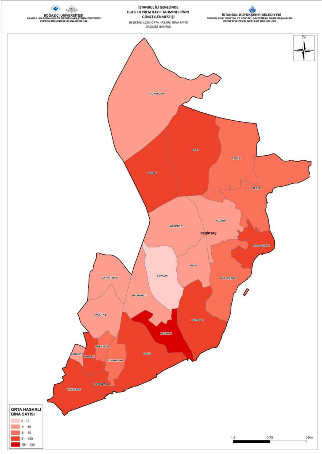
Şekil 5-4: Mw=7.5 Senaryo Depremi İçin Beşiktaş İlçesi Tahmini Orta Hasarlı Bina Sayısı Dağılım Haritası
