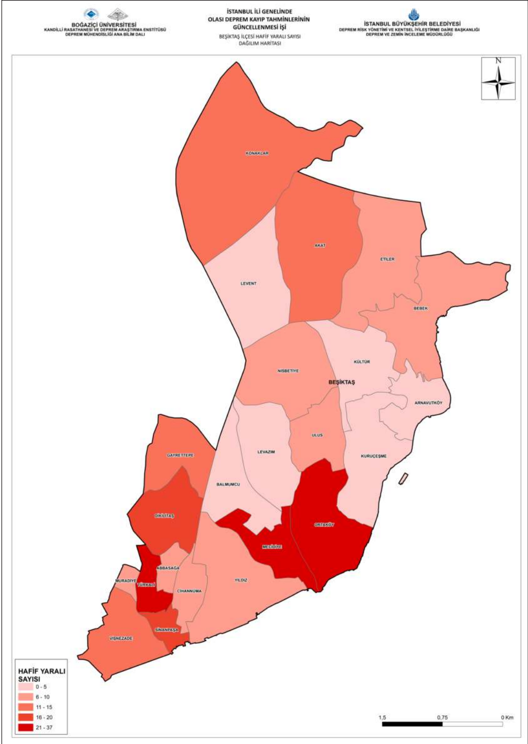
Şekil 5-6: Mw=7.5 Gece Senaryosu Depremi İçin Beşiktaş İlçesi Tahmini Hafif Yaralı Sayısı Dağılım Haritası
